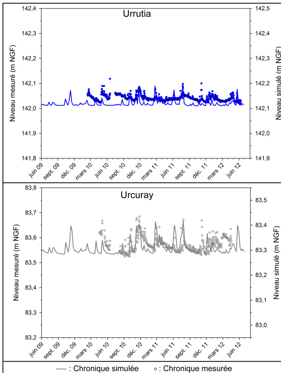
Figure IV-19. Niveaux observés et simulés dans les cours d'eau Urrutia et Urcuray
