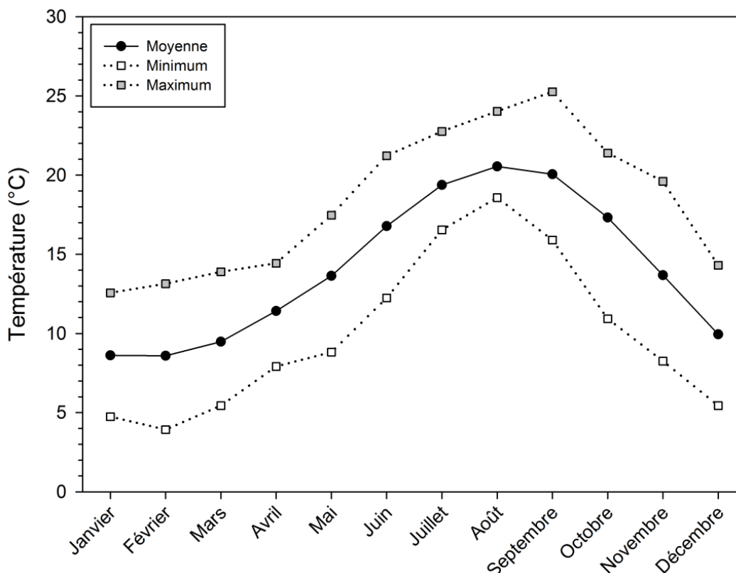
Figure I-10. Températures mensuelles moyennes, minimums et maximums enregistrés à Cambo-les-Bains entre 1964 et 2009
