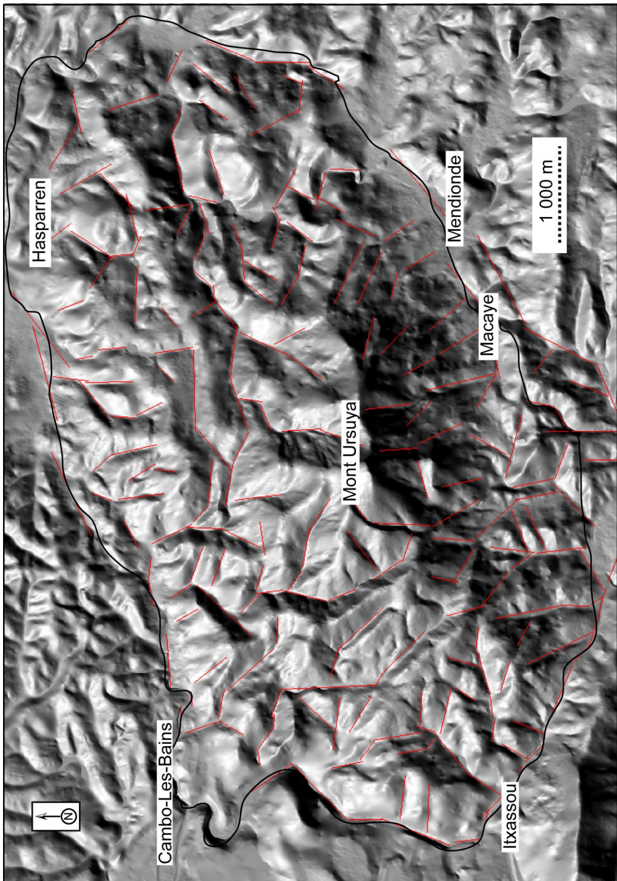
Figure I-13. MNT (éclairage azimuth 315°) et linéaments répertoriés
